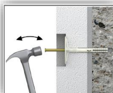
3. Montaj diblu
